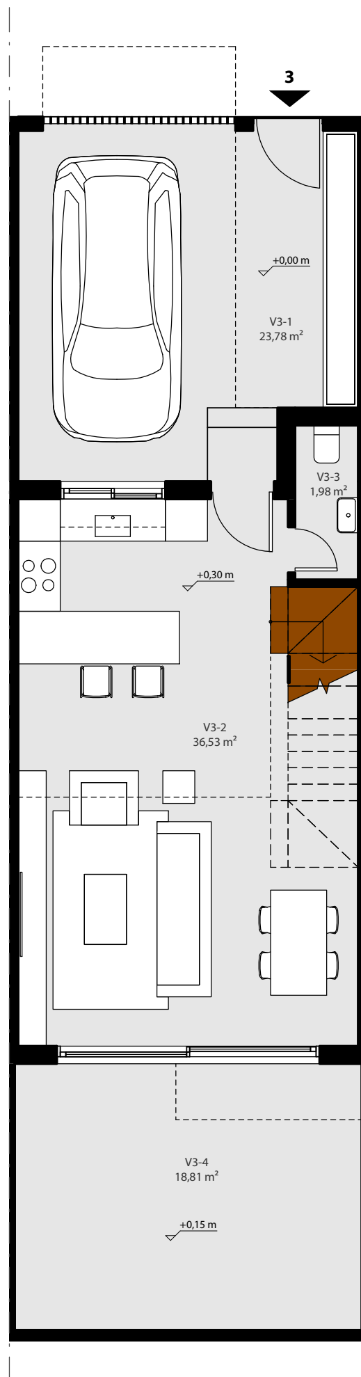
0 Planta Baja 09 1 : 75
