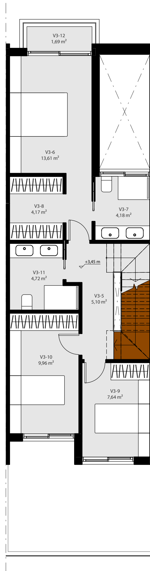
1 Planta Primera 09 1 : 75
