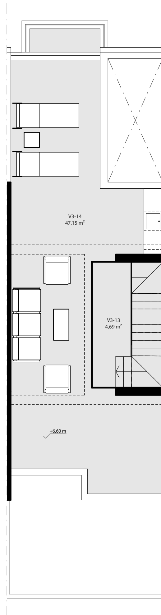
2 Planta Segunda 09 1 : 75
