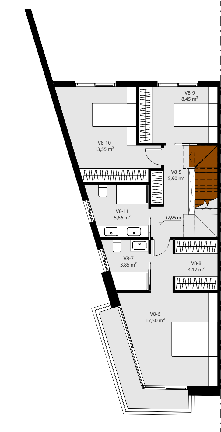
1 Planta Primera 14 1 : 100
