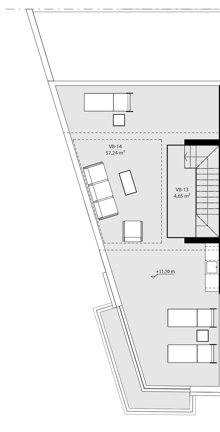
2 Planta Segunda 14 1 : 100
