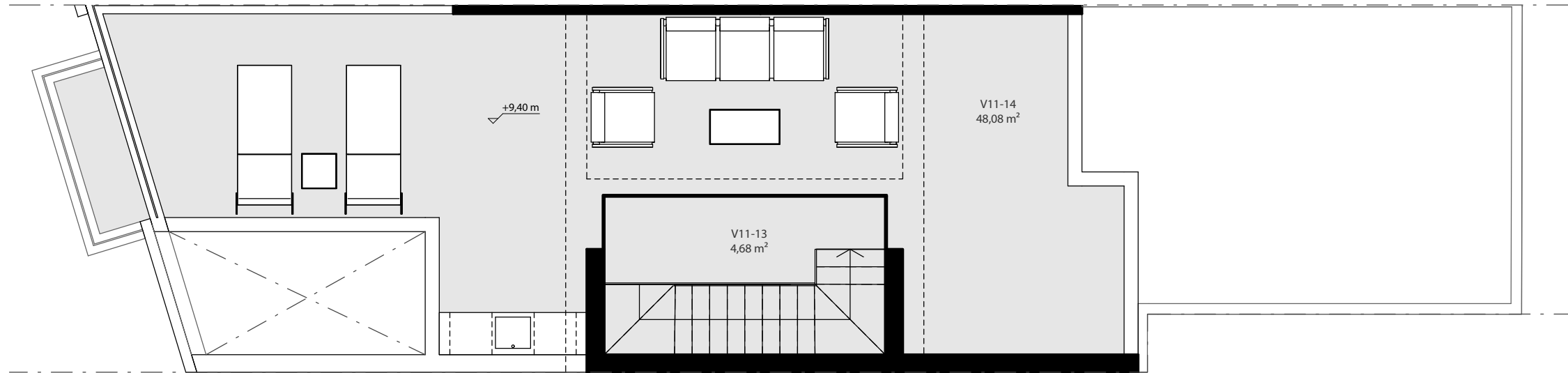
2 Planta Segunda 17 1:75
