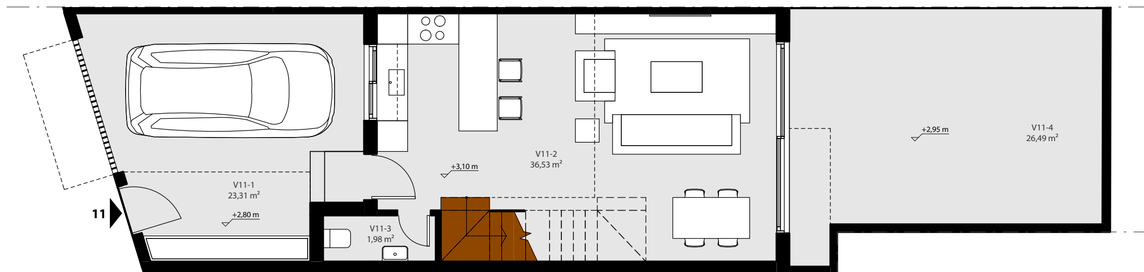
0 Planta Baja 17 1:75
